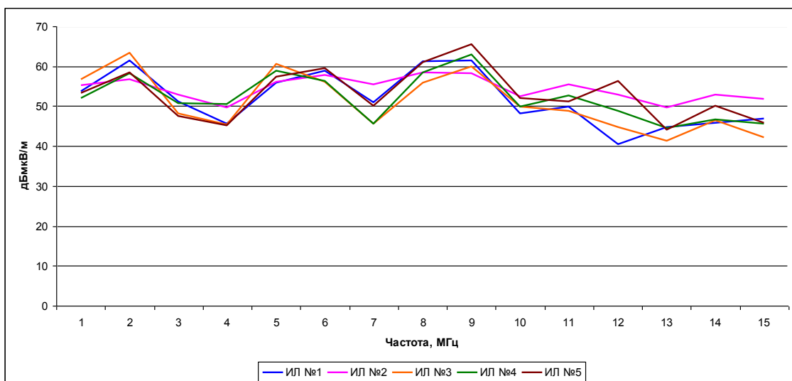
Рисунок 8. График измерений мощности радиопомех.
