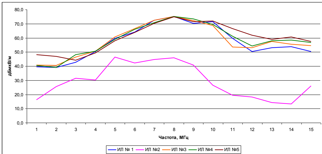
Рисунок 1. График измерений напряженности поля радиопомех при горизонтальной поляризации.
