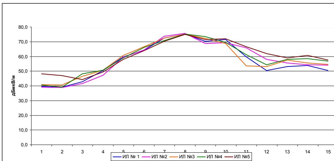
Рисунок 5. График измерений напряженности поля радиопомех при горизонтальной поляризации.
