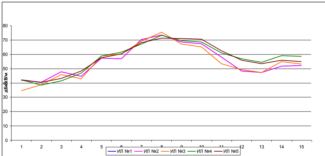
Рисунок 6. График измерений напряженности поля радиопомех при вертикальной поляризации.
