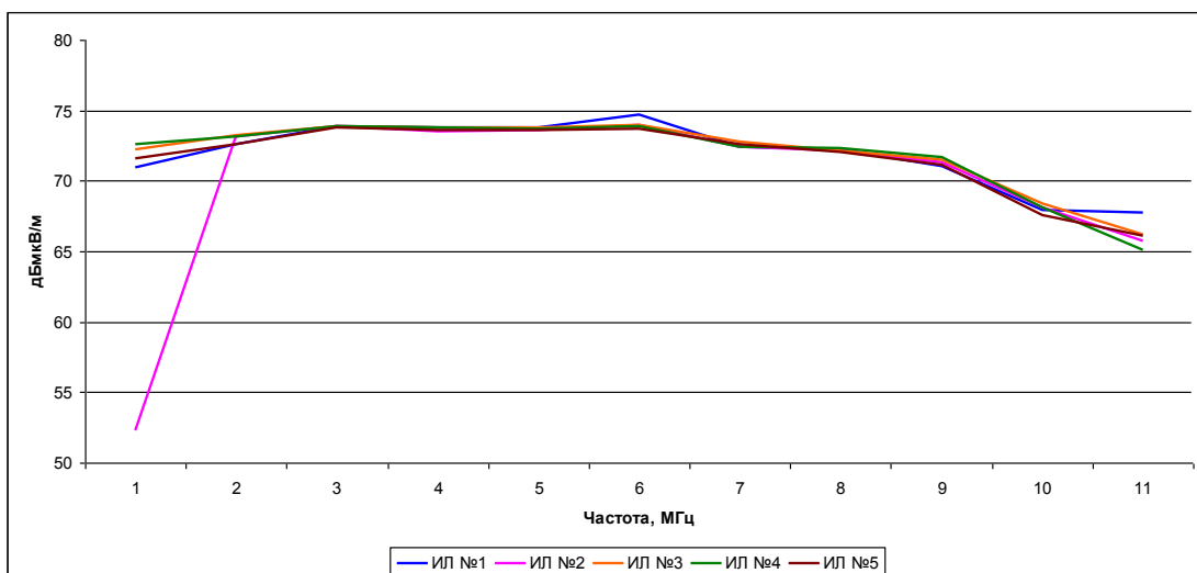
Рисунок 2. График измерений напряженности поля радиопомех при вертикальной поляризации.
