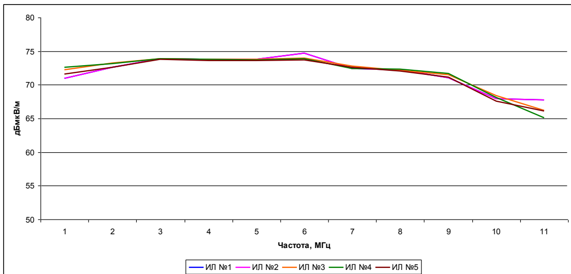
Рисунок 7. График измерений несимметричного напряжения радиопомех.
