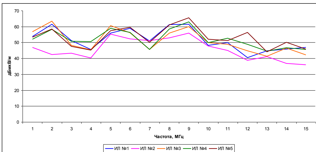
Рисунок 4. График измерений мощности радиопомех.
